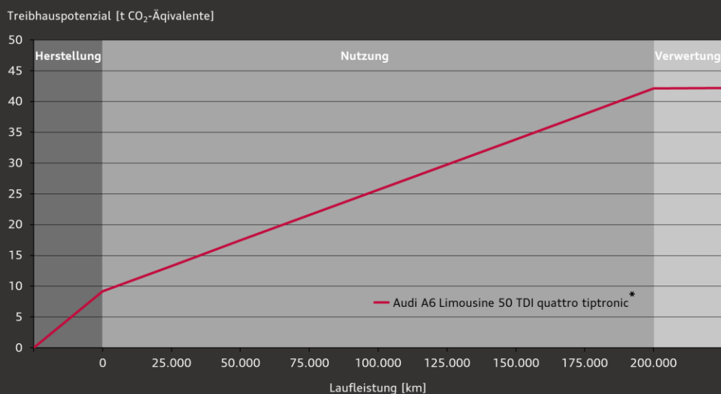
Abbildung 2: Treibhauspotenzial des Audi A6 Limousine 50 TDI quattro tiptronic* über den gesamten Lebenszyklus
